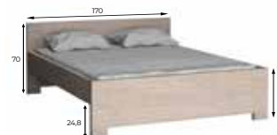
V-19 A 170/B 210/70 pod materac 160 x 200
